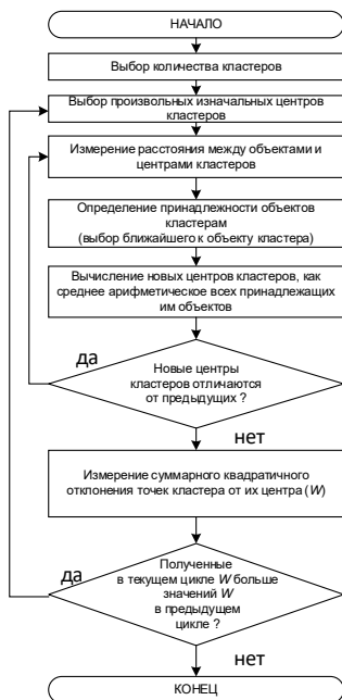
Рис. 2. Алгоритм метода k-средних
