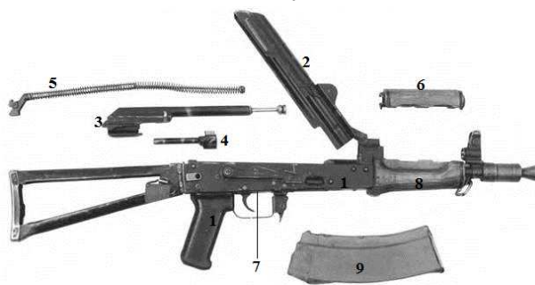
АКС-74У
