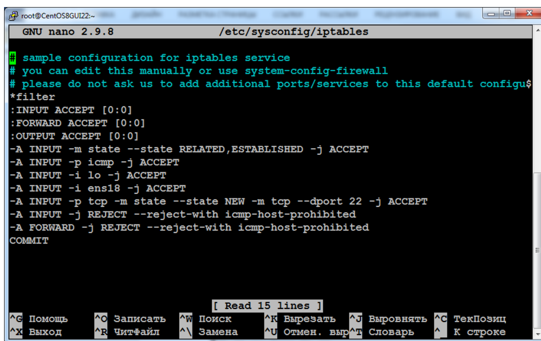
Рис. 3.2.3. Вид конфигурационного файла межсетевого экран-маршрутизатора iptables в ОС CentOS8
