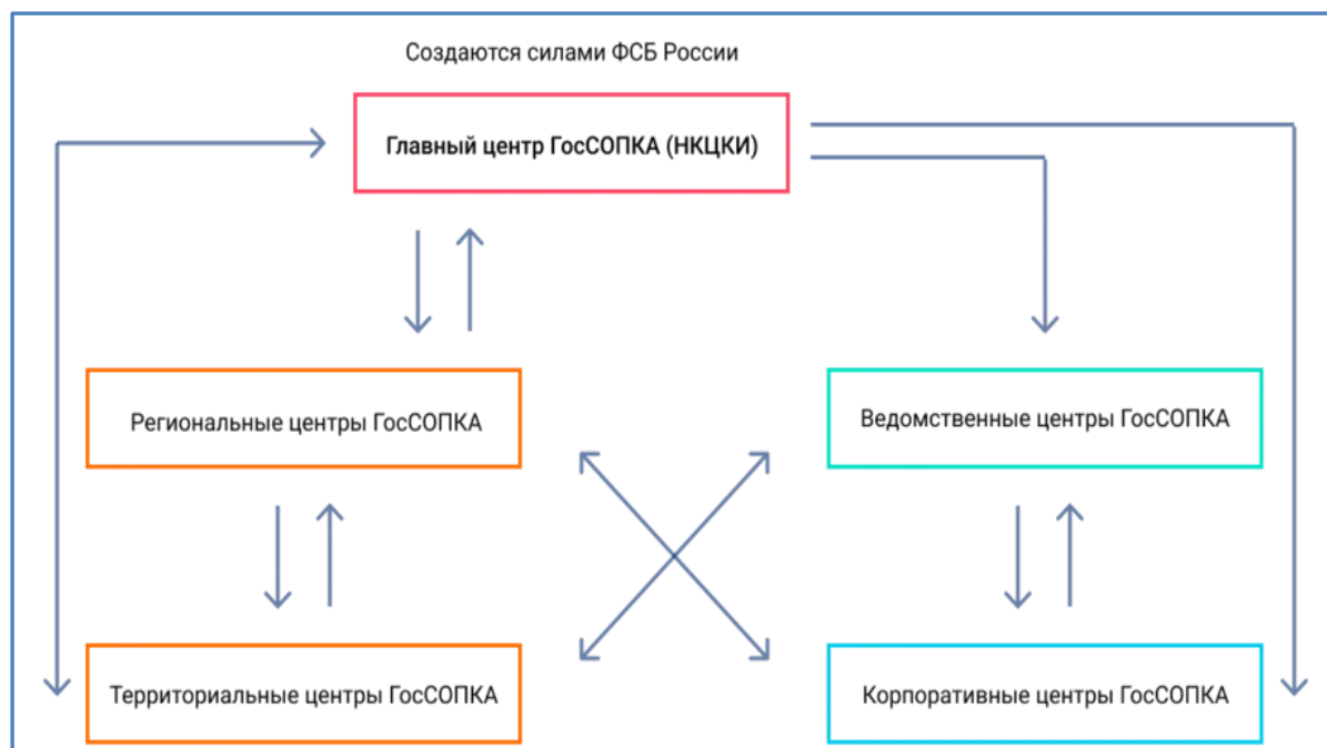
Рис. 2.4.1. Организационная структура ГосСОПКА
