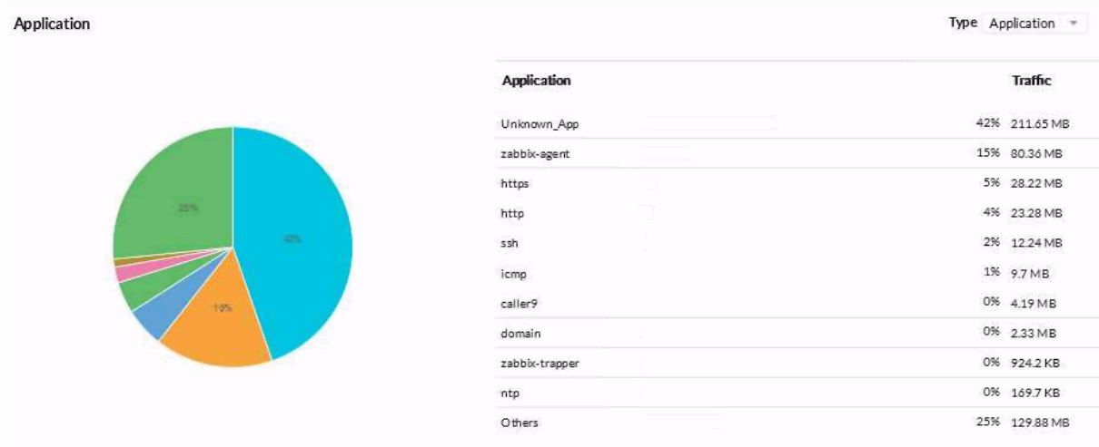
Рис. 6.5.8. Распределение объемов переданной информации по видам приложений
