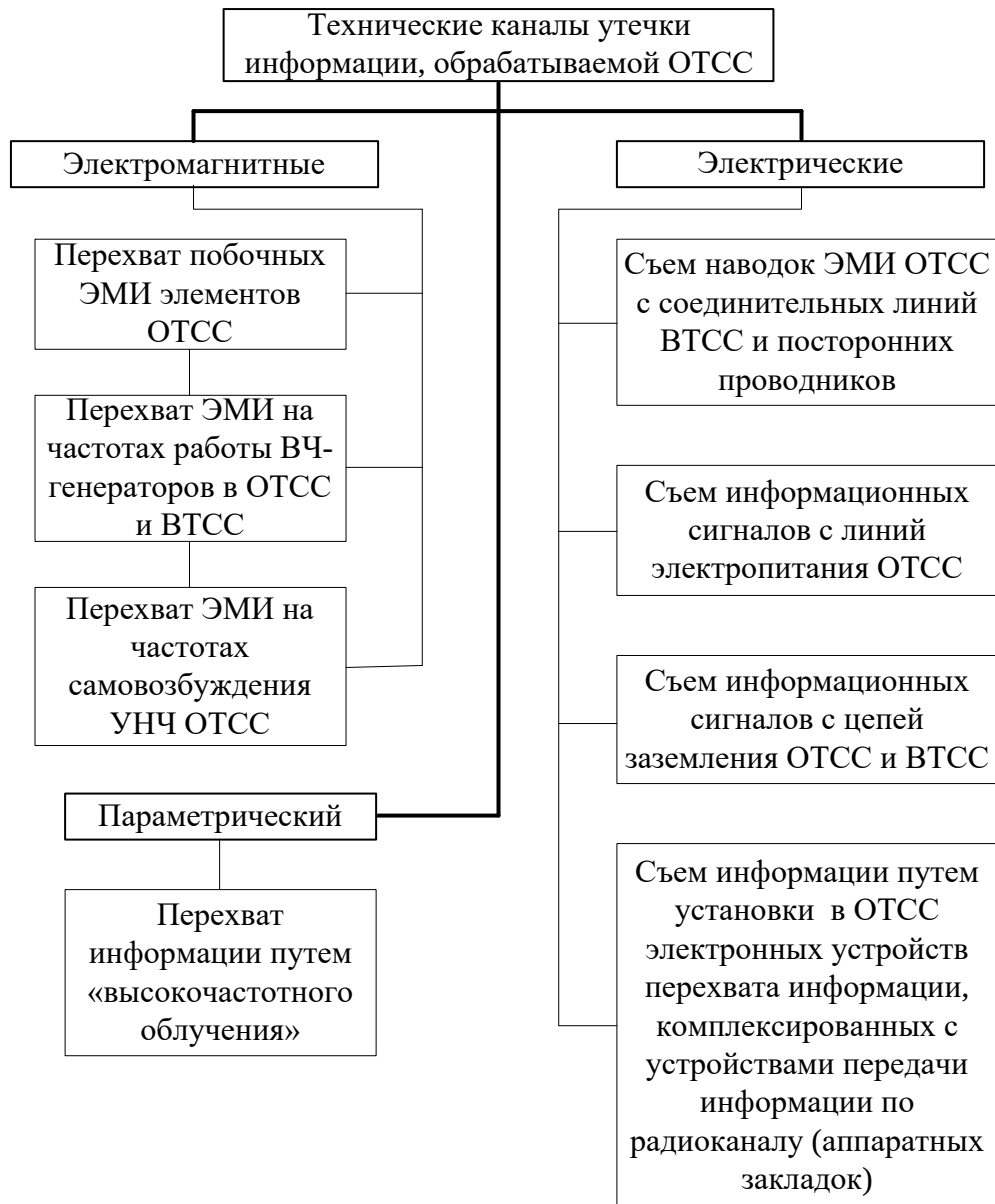
Рис. 4.1.1. Классификация технических каналов утечки информации, обрабатываемой ТСПИ
