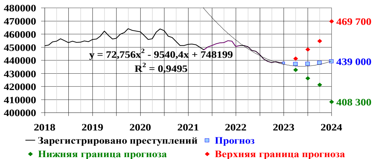
Рис. 3.2. Динамика и прогноз числа зарегистрированных преступлений в Центральном федеральном округе
