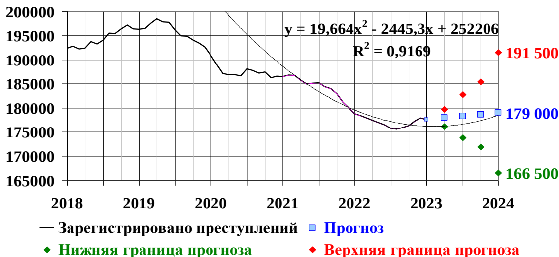
Рис. 3.6. Динамика и прогноз числа зарегистрированных преступлений в Уральском федеральном округе
