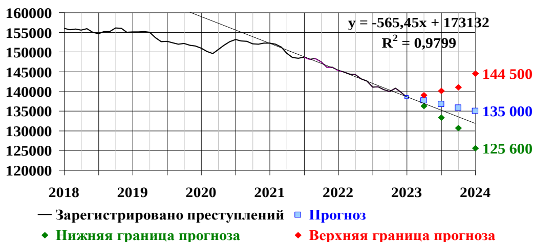
Рис. 3.8. Динамика и прогноз числа зарегистрированных преступлений в Дальневосточном федеральном округе
