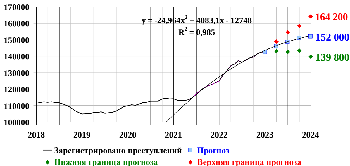
Рис. 3.10. Динамика и прогноз числа зарегистрированных особо тяжких преступлений
