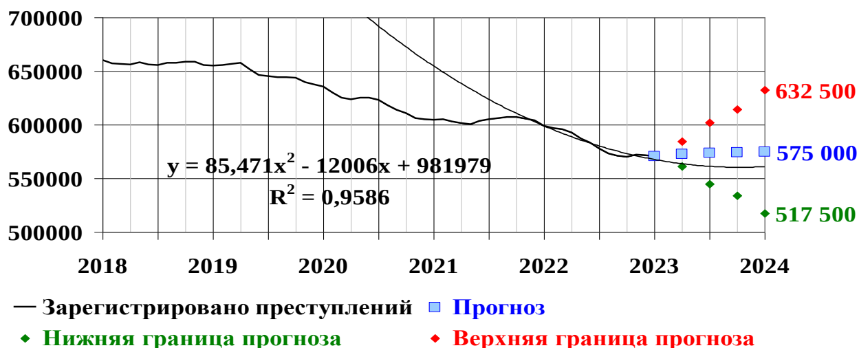
Рис. 3.12. Динамика и прогноз числа зарегистрированных преступлений средней тяжести
