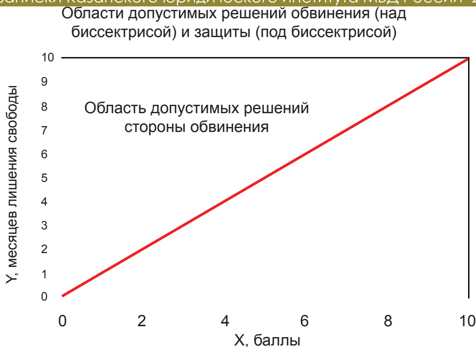
Рис. 2. Области допустимых решений сторон обвинения (подписано – «область допустимых решений стороны обвинения») и защиты (без подписи), разделенные линией биссектрисы.
