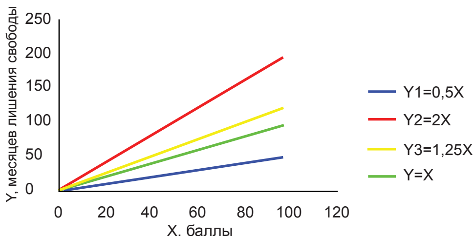
Рис. 1. Функции защиты, обвинения, равновесного и биссекториального приговоров по уголовному делу о разбойном нападении.
