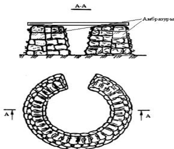
Рис. 7. Сооружение для ведения огня из мешков с песком
