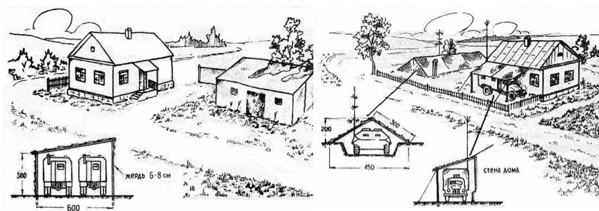
Рис. 14. Варианты маскировки техники в населенном пункте
