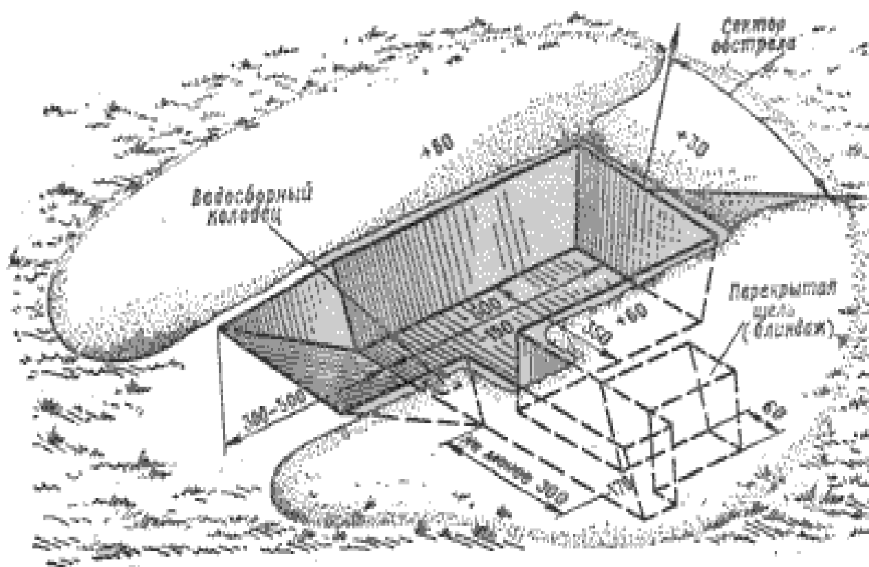
Рис. 31 Окоп для бронетранспортера
