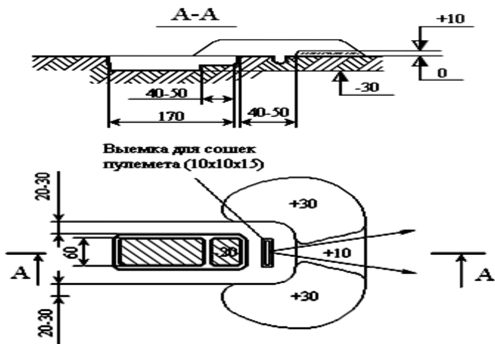
Рис.2. Окоп для стрельбы из пулемета лежа Объем вынутого грунта 0,3 \text{ м}^3 . На устройство окопа пехотной
