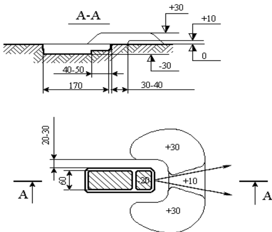
Рис.1. Окоп для стрельбы из автомата лежа
