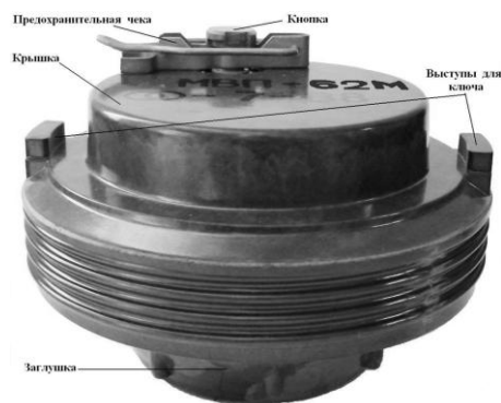
Рис. 21. Взрыватель МВП-62М
