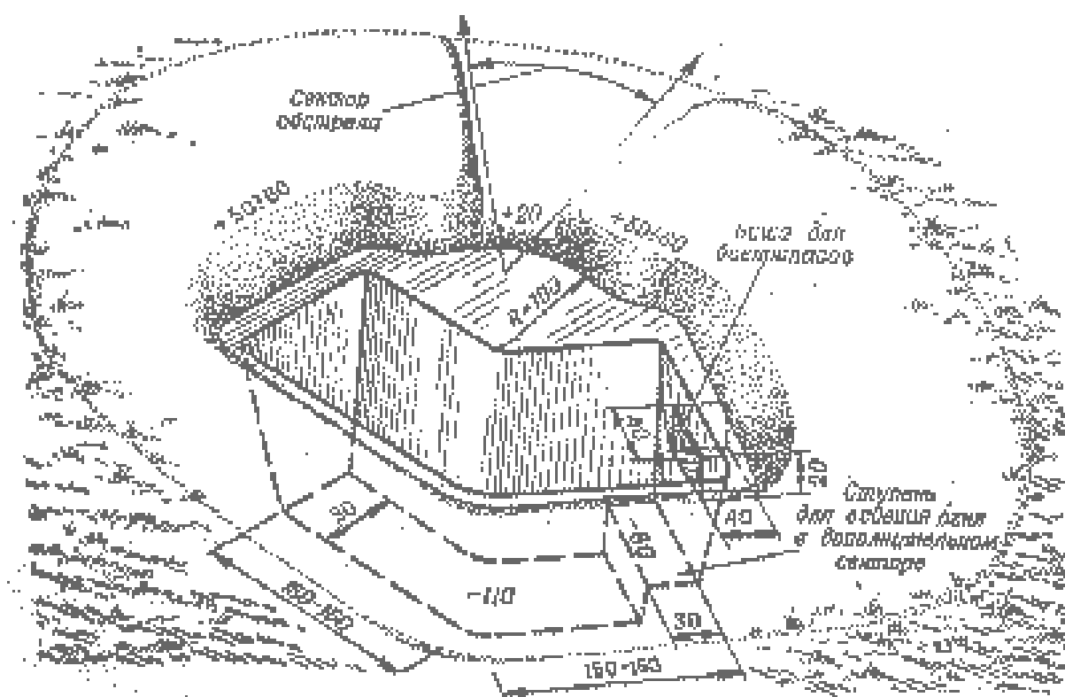
Рис. 30 Окоп для стрельбы из пулемета стоя
