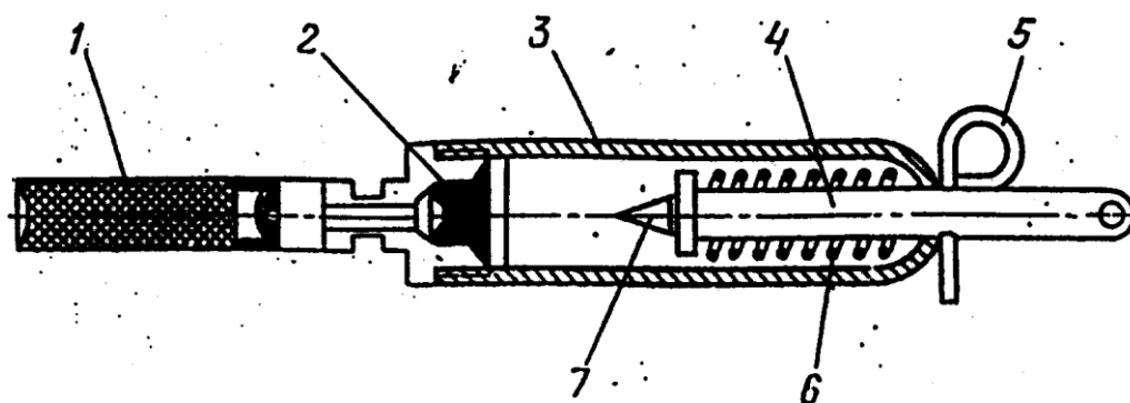
Рис. 17. Минный универсальный взрыватель (МУВ).
