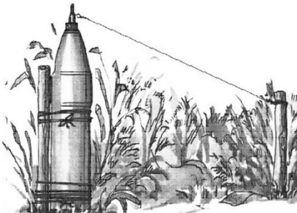
Рис. 23. Вариант использования осколочно-фугасного снаряда в качестве «Фугаса» с применением взрывателя МУВ и растяжки-шнура
