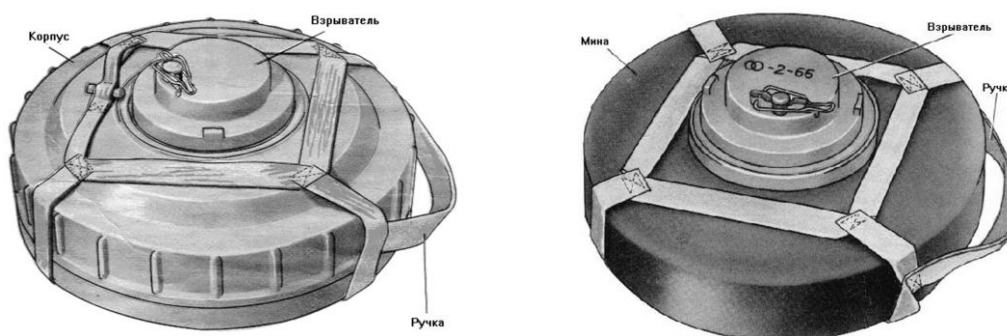
Рис. 22. Противотанковые мины ТМ-62П2 и ТМ-62Т
