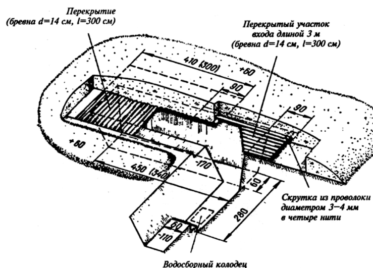
Рис. 8. Перекрытая щель на отделение
