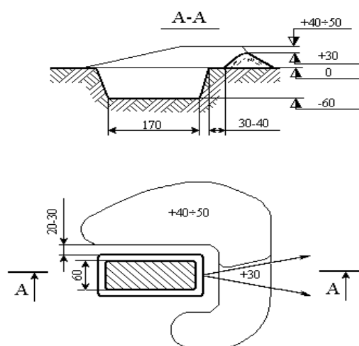
Рис. 28. Окоп для стрельбы из автомата с колена
