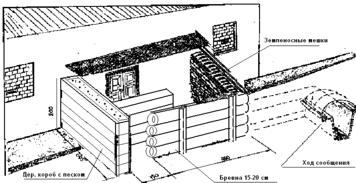
Рис. 10. Защищенный вход в здание
