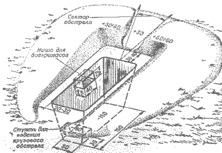
Рис. 29. Окоп для стрельбы из автомата стоя: 1 – ступень для ведения кругового обстрела; 2 – ниша для боеприпасов
