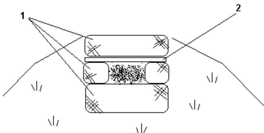
Рис. 4. Устройство амбразуры из мешков с песком: 1 – мешки с песком, 2 – доска
