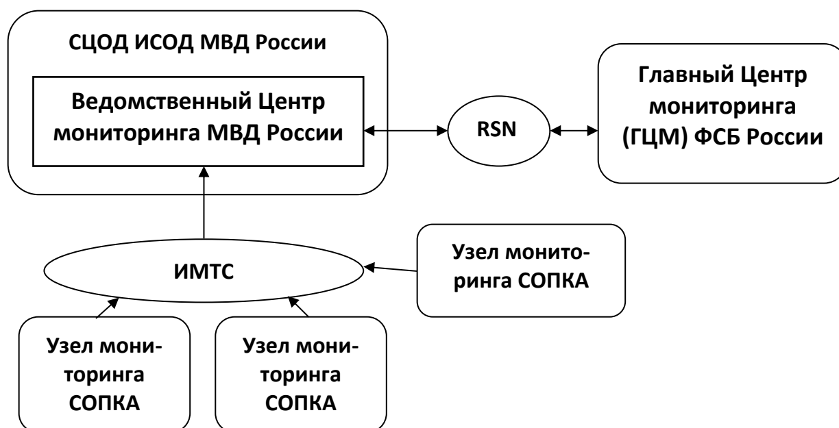
Рис. 11. Структура СОПКА МВД России
