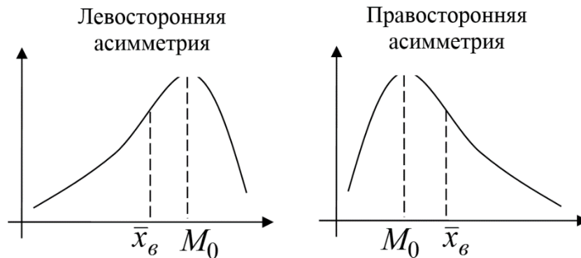
Рис. 18.4. Левосторонняя и правосторонняя асимметрии.
