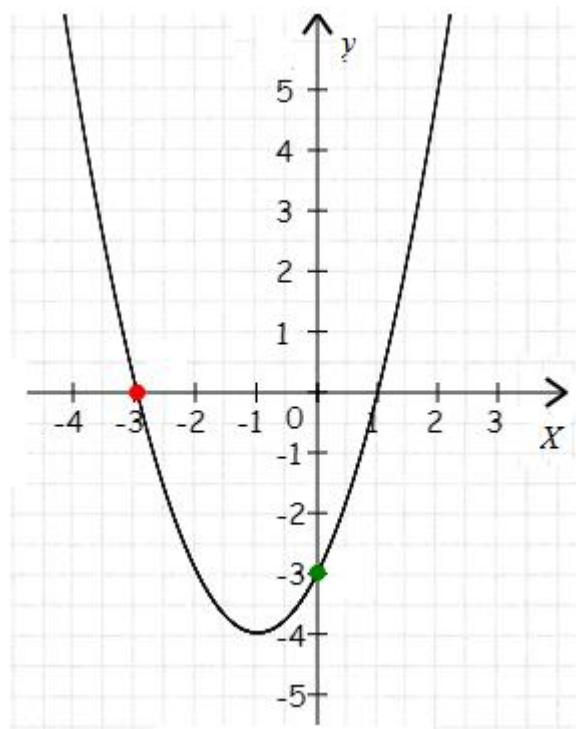
Рис. 9.5. График функции y = x^2 + 2x - 3 .
