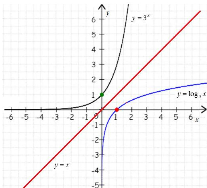
Рис. 9.8. Графики функций y = 3^x и y = \log_3 x .
