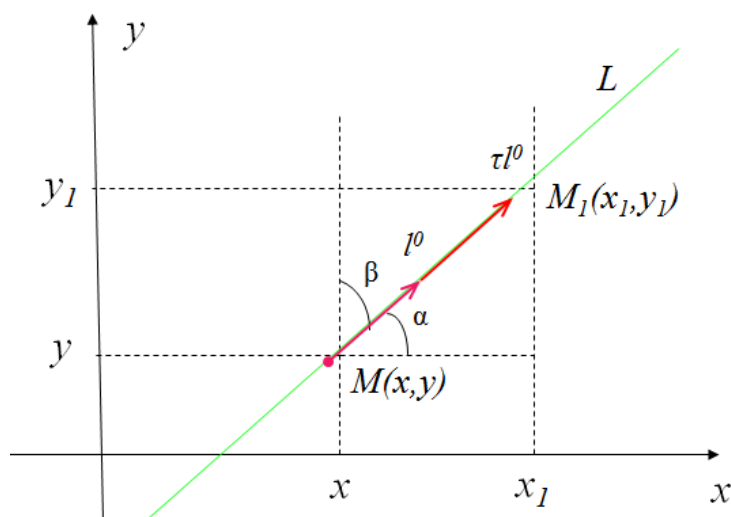
Рис. 11.3. Производная по направлению.
