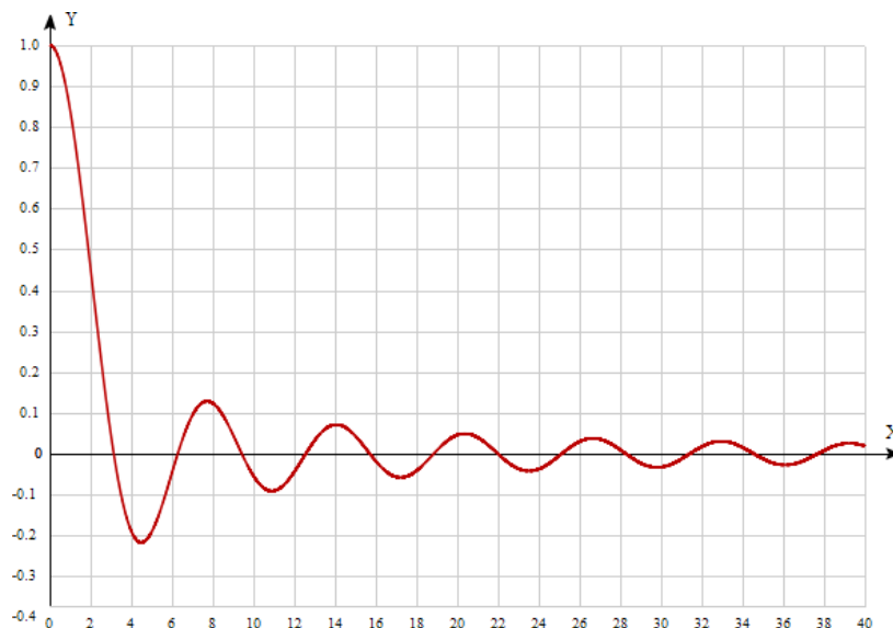
Рис. 10.4. График функции y = \frac{\sin x}{x} .
