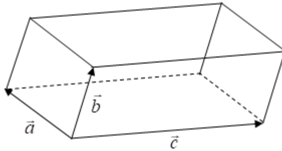
Рис. 3.12. Геометрическое представление смешанного произведения.
