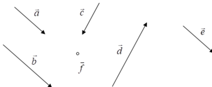
Рис. 3.3. Коллинеарные и равные векторы.
