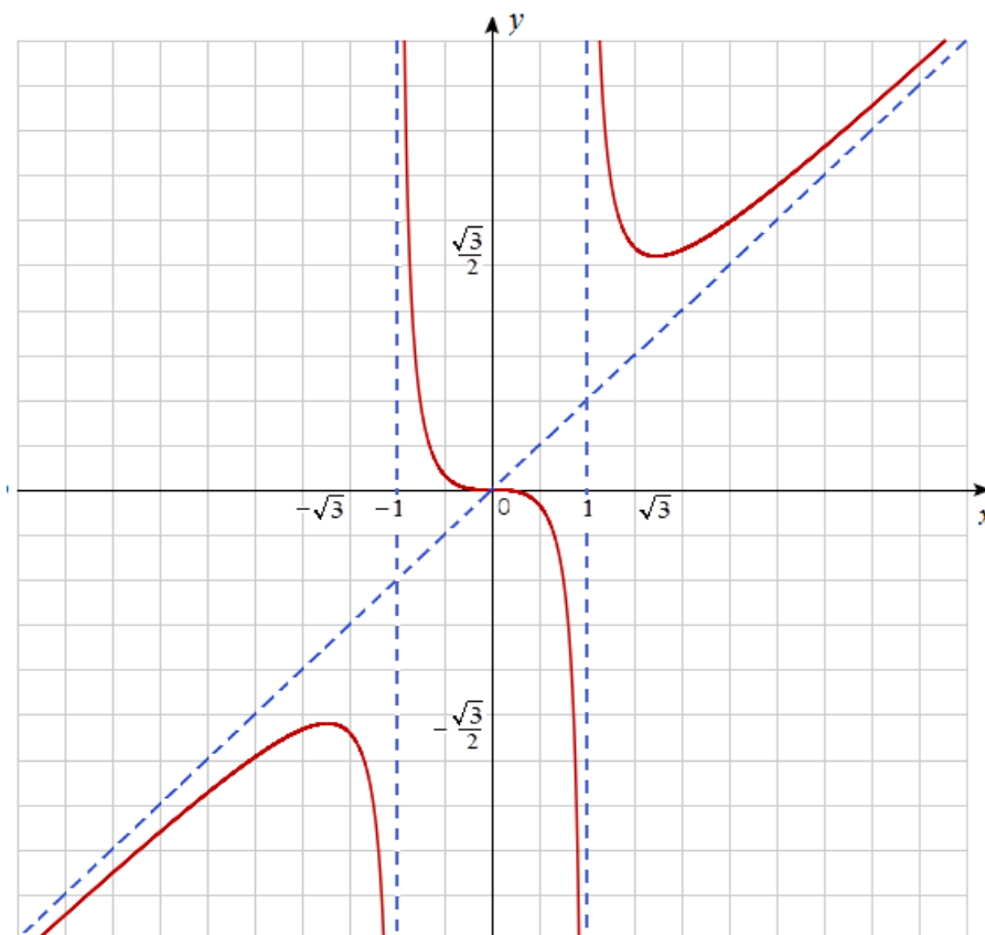
Рис. 10.18. График функции f(x) = \frac{x^3}{x^2 - 1} .
