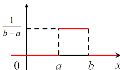
Рис. 17.3. График плотности распределения случайной величины, имеющей равномерный закон распределения.
