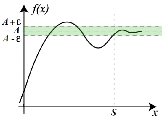
Рис. 9.10. Геометрический смысл предела функции в бесконечности.
