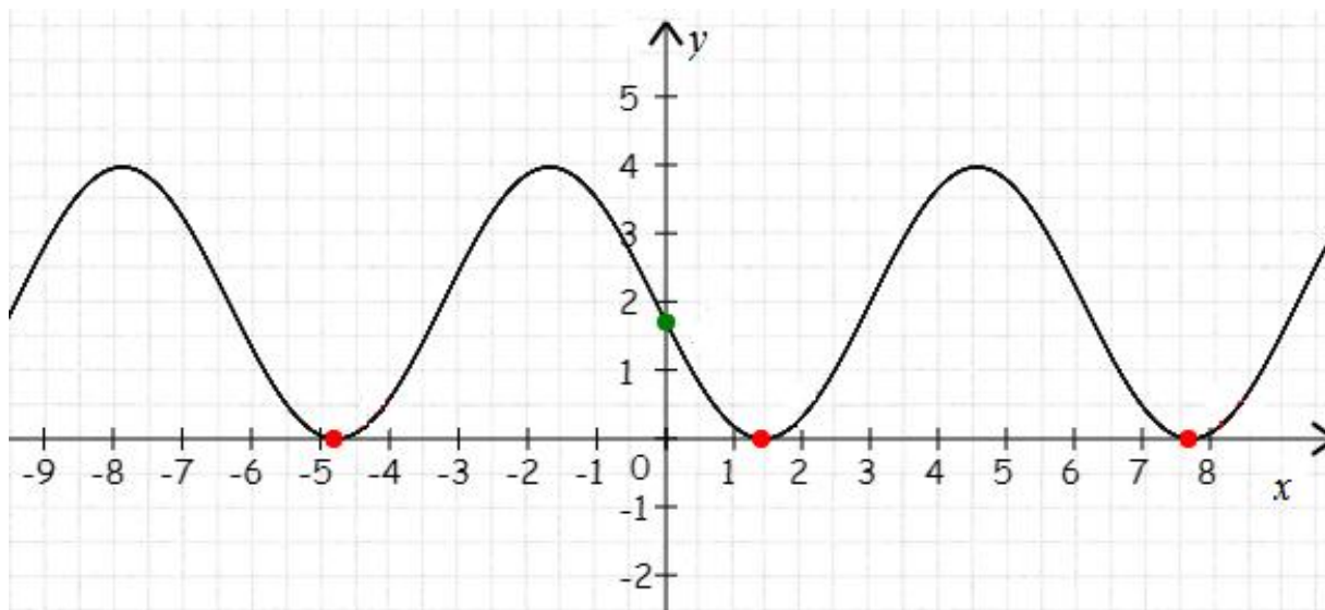
Рис. 9.6. График функции y = 2\sin(x - 3) + 2 .
