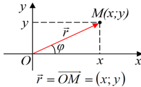
Рис. 6.2. Графическое изображение комплексного числа.
