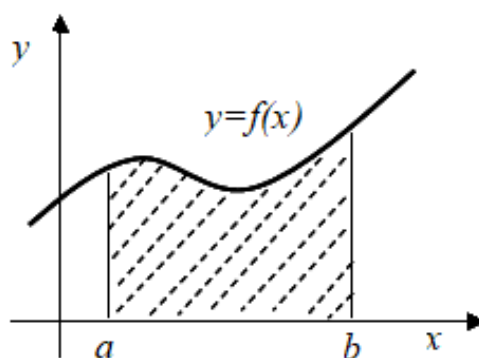
Рис. 12.3. Нахождение площади криволинейной трапеция.
