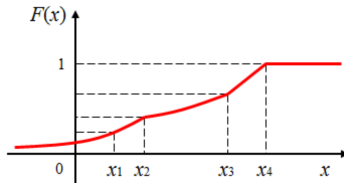
Рис.17.1. График функции распределения непрерывной случайной величины.
