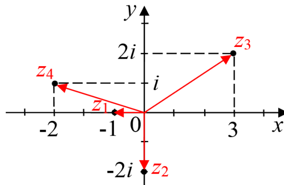
Рис. 6.3. Изображение чисел -1 ; -2i ; 3 + 2i ; -2 + i .
