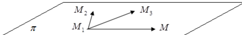
Рис. 4.3. Плоскость, проходящая через три точки.
