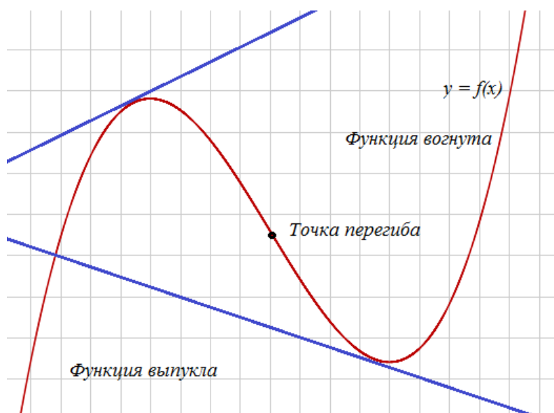
Рис. 10.5. Выпуклость и вогнутость функции.
