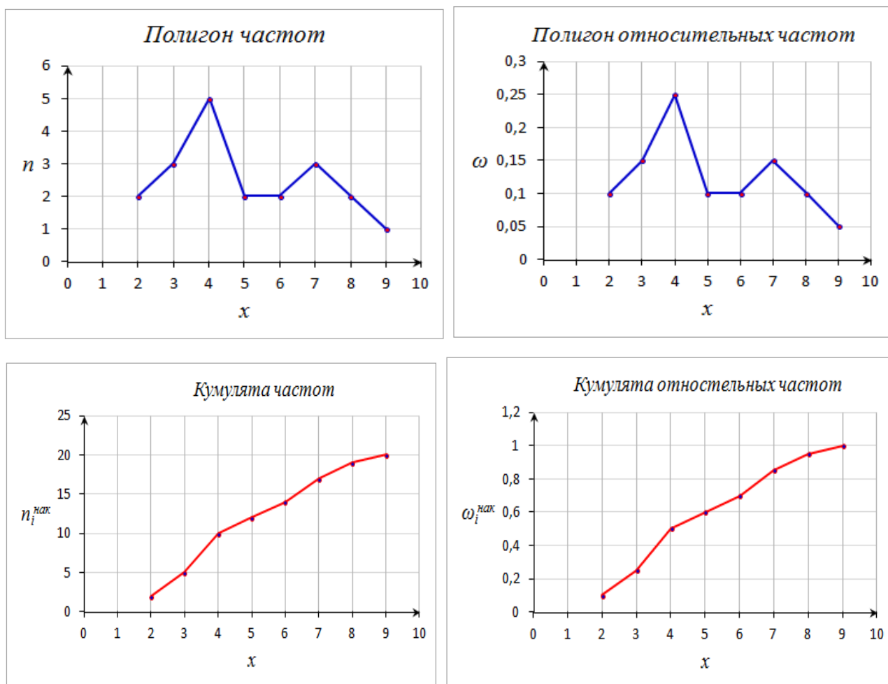
Рис. 18.2. Графическое представление дискретного вариационного ряда.
