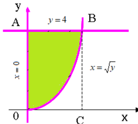
Рис. 12.7. Площадь криволинейного треугольника.
