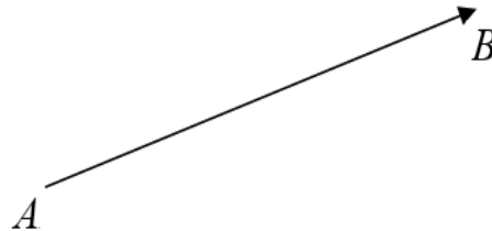
Рис. 3.1. Геометрическое изображение вектора.
