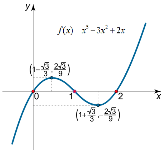
Рис. 10.7. График функции f(x) = x^3 - 3x^2 + 2x .
