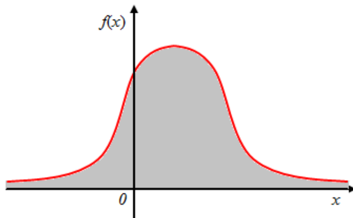
Рис. 17.2. Площадь фигуры, ограниченной осью Ox , кривой распределения f(x)
