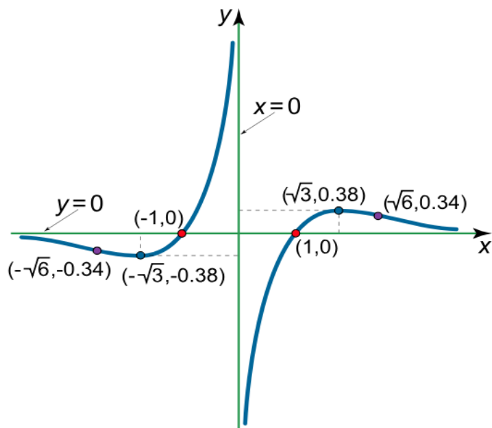
Рис 10.13. График функции f(x) = \frac{x^2 - 1}{x^3} .
