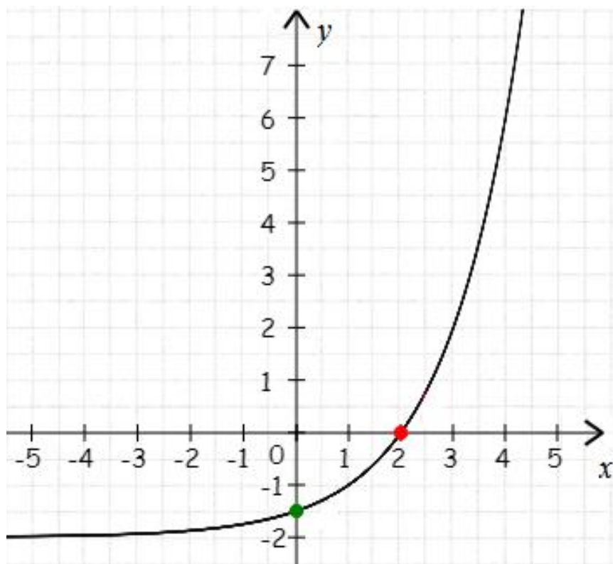
Рис. 9.7. График функции y = 2^{x-1} - 2 .
