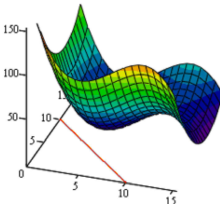
Рис. 11.5. Функция двух переменных.
