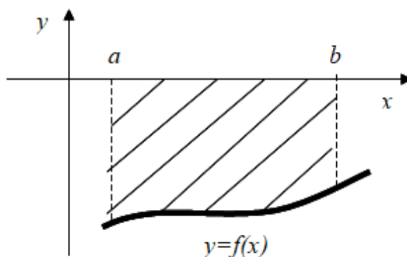
Рис. 12.5. Случай неположительной функции y = f(x) .
