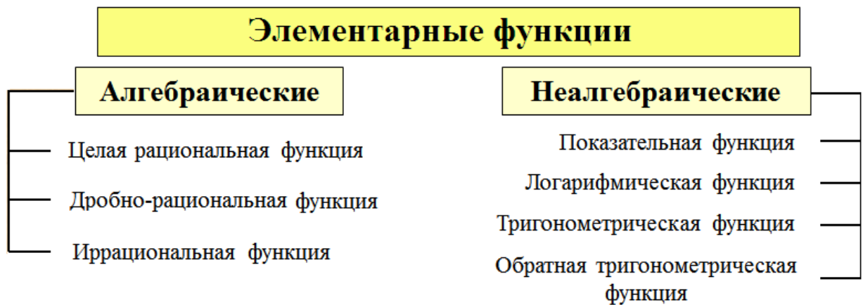
Рис. 9.9. Классификация элементарных функций.
