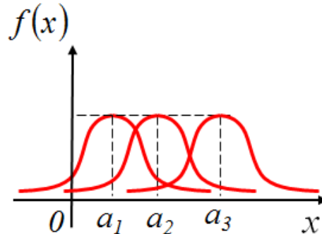
Рис. 17.7. Влияние параметра a на форму нормальной кривой.
