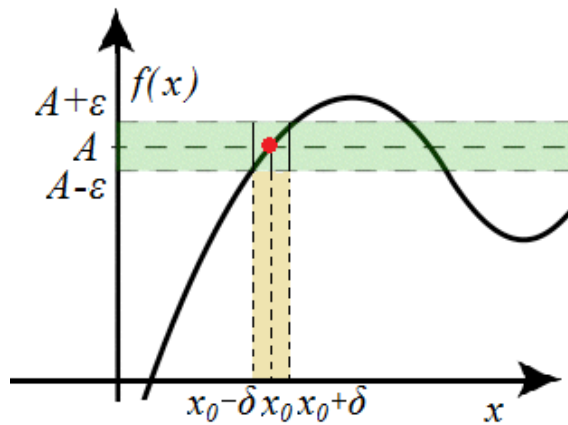
Рис. 9.12. Геометрический смысл предела функции в точке.
