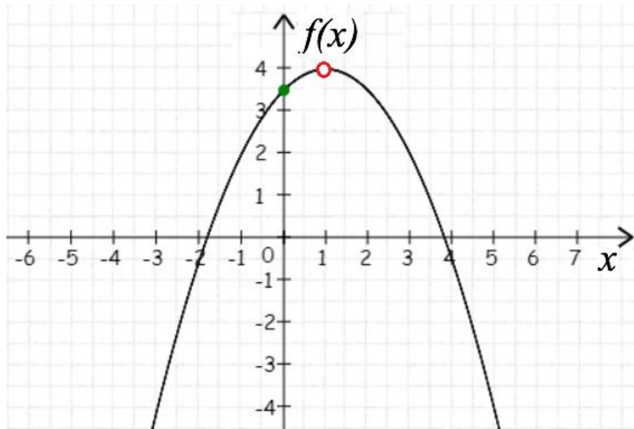
Рис. 9.13. График функции f(x) = \frac{-(x-1)^3}{2x-2} + 4 .
