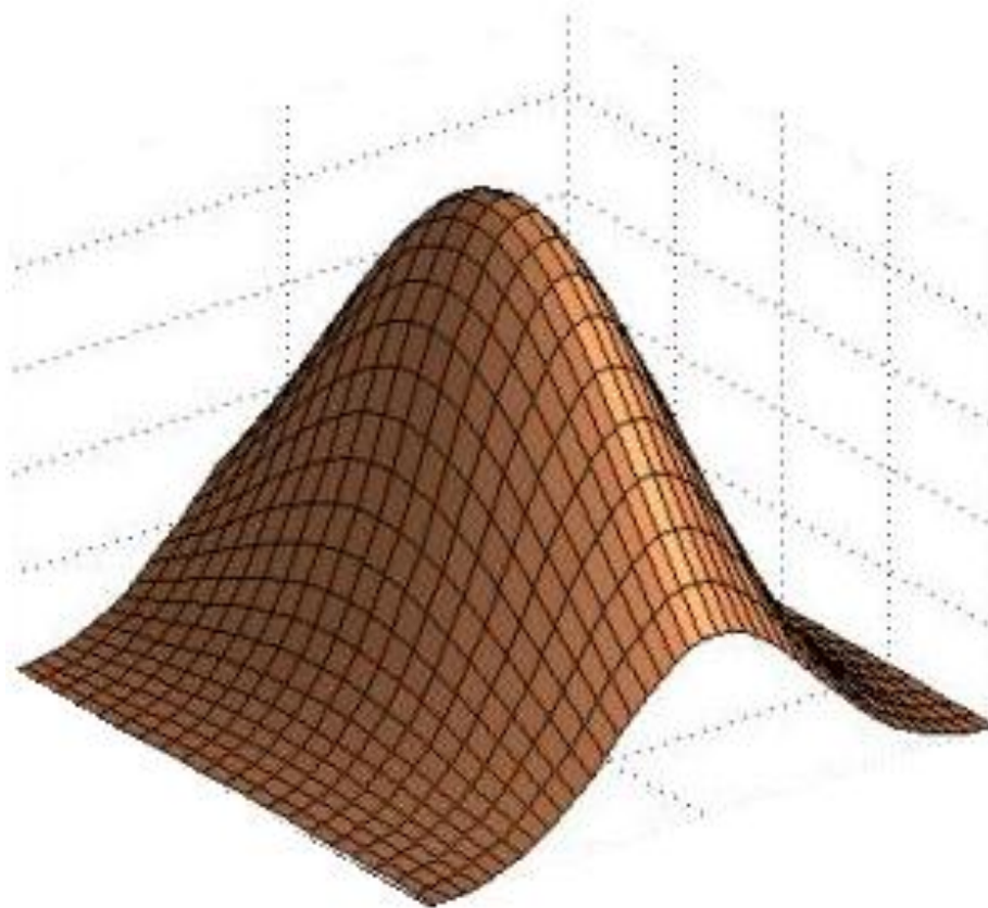
Рис. 11.2. График функции, непрерывной в прямоугольной области.
