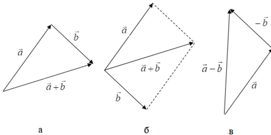
Рис. 3.5. Сумма и разность векторов.
