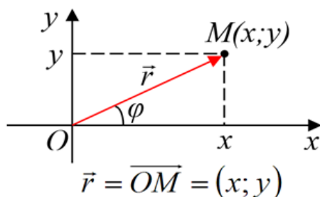
Рис. 6.4. Модуль и аргумент комплексного числа.
