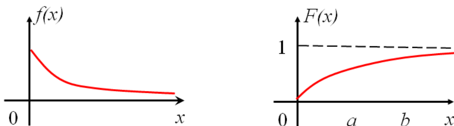
Рис. 17.5. Графики плотности распределения и функции распределения случайной величины, имеющей показательный закон распределения.
