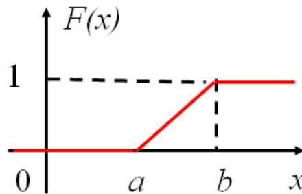
Рис. 17.4. График функции распределения случайной величины, имеющей равномерный закон распределения.
