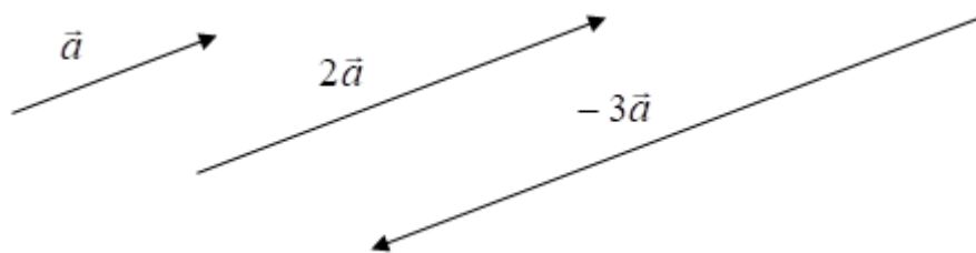
Рис. 3.6. Умножение вектора на число.
