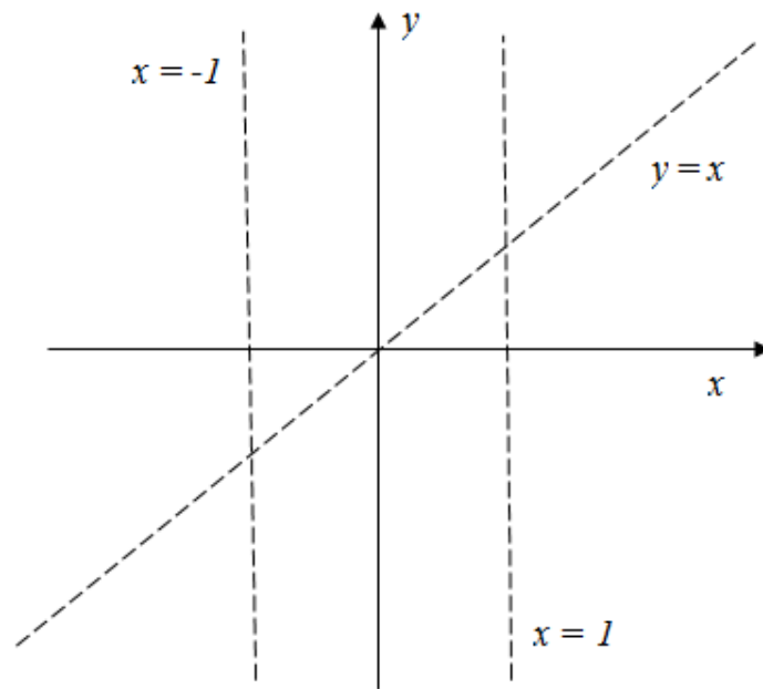
Рис. 10.15. Асимптоты исследуемой функции.
