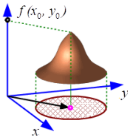
Рис. 11.4. Максимум функции двух переменных.
