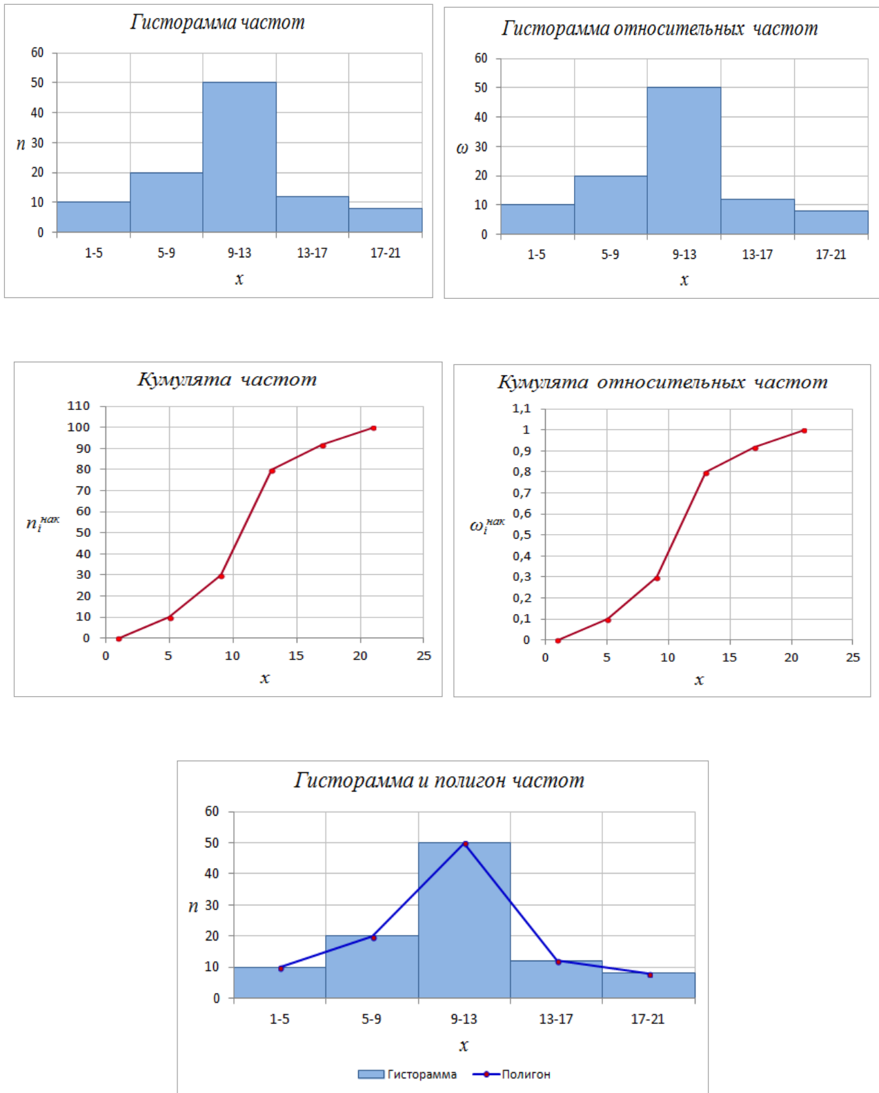
Рис. 18.3. Графическое представление интервального вариационного ряда.
