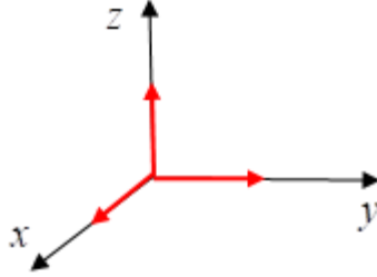
Рис. 3.11. Орты осей координат.
