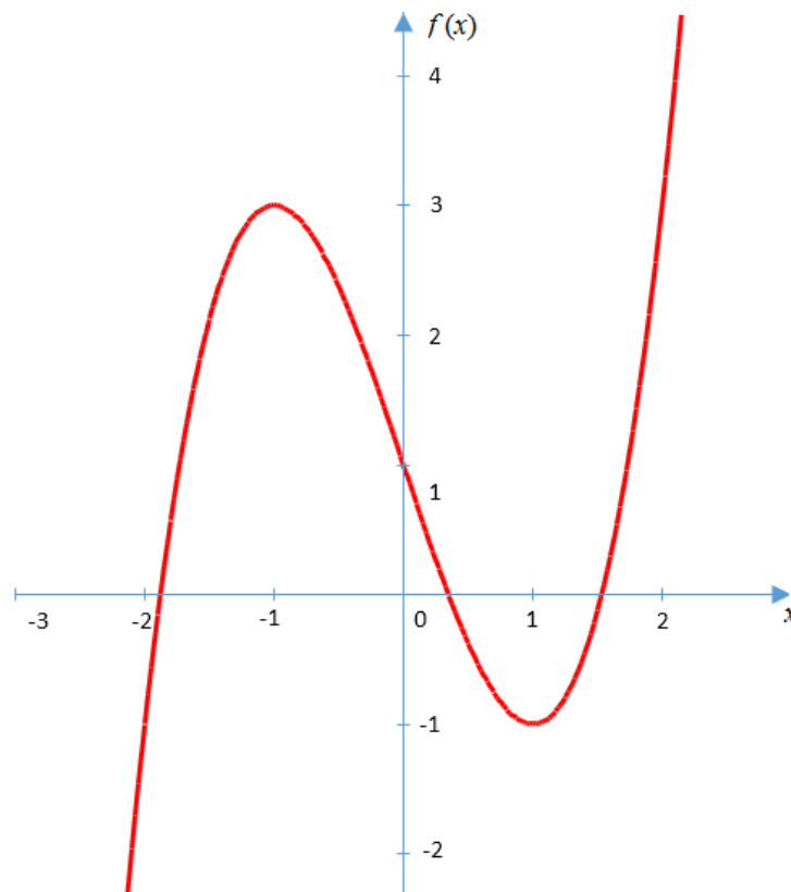
Рис. 10.2 График функции f(x) = x^3 - 3x + 1 .
