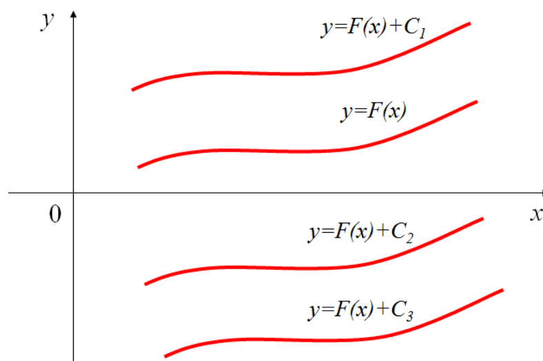
Рис. 12.1. Семейство кривых F(x) + C .
