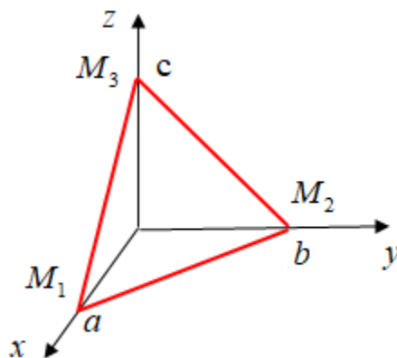
Рис. 4.4. Пересечение плоскости \pi с осями координат.
