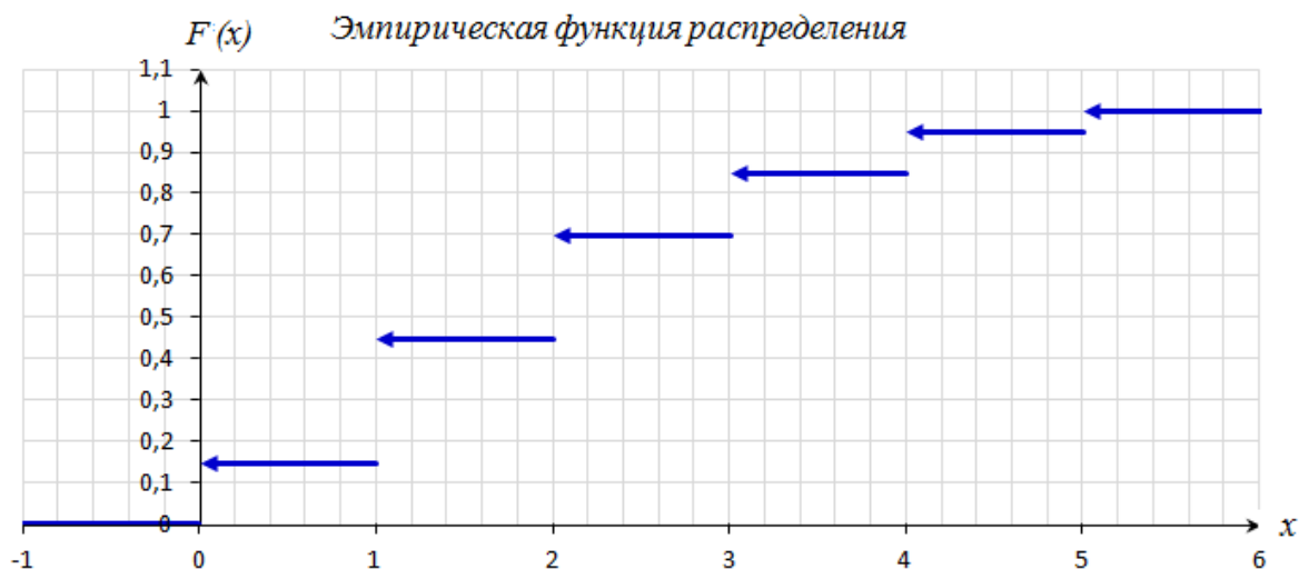
Рис. 18.1. Эмпирическая функция распределения.
