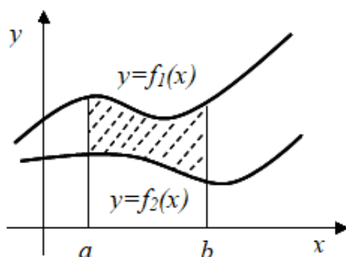
Рис. 12.4. Площадь фигуры, ограниченная кривыми y=f_1(x) и y=f_2(x) .
