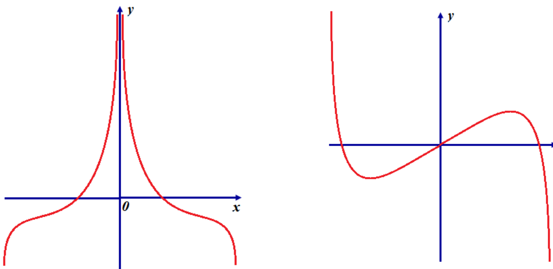
Рис. 9.4. Графики четной (слева) и нечетной (справа) функций.
