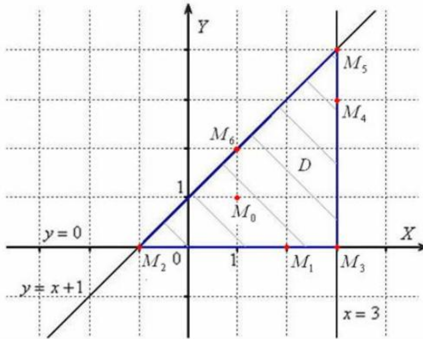
Рис. 11.6. Область определения функции.
