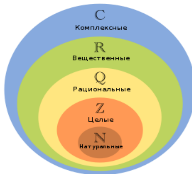
Рис. 6.1 Множество комплексных чисел.
