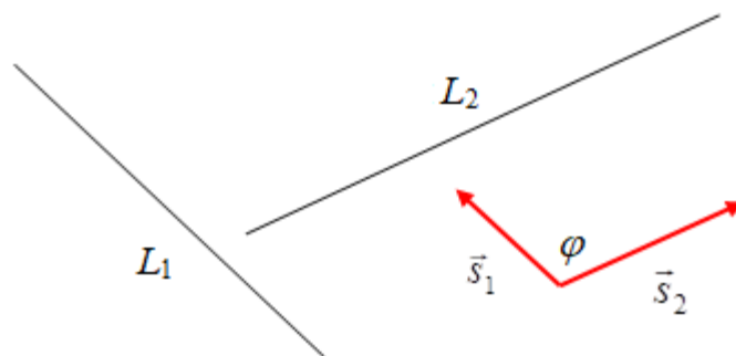
Рис.4.8. Угол между прямыми.
