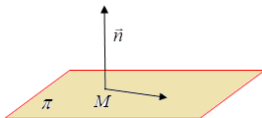
Рис. 4.1. Определение общего уравнения.
