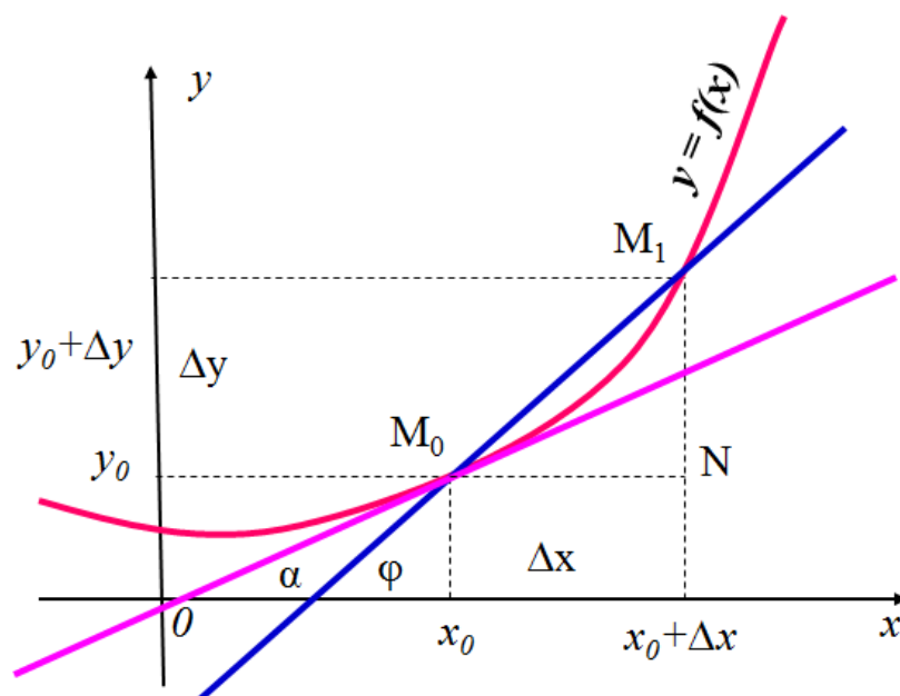
Рис. 10.1. Геометрический смысл производной.
