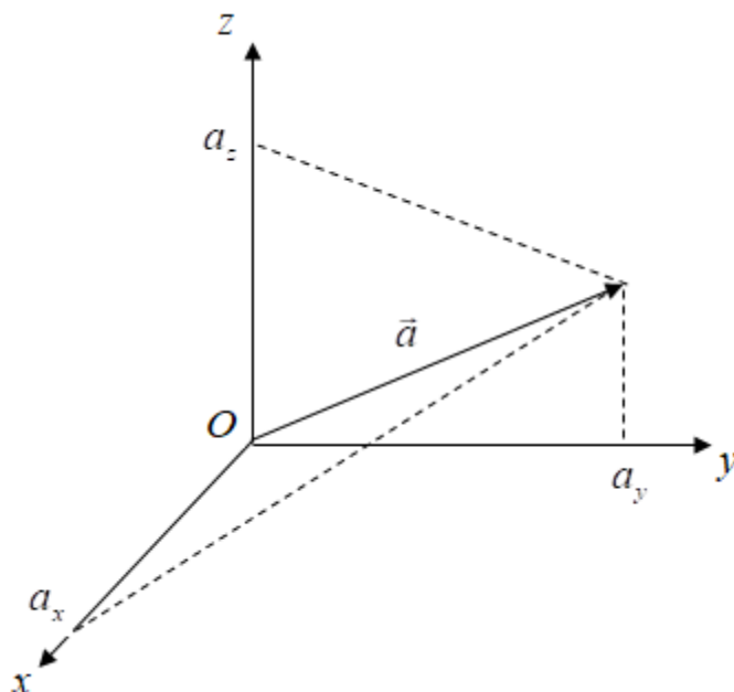
Рис. 3.7. Проекция вектора \vec{a} .
