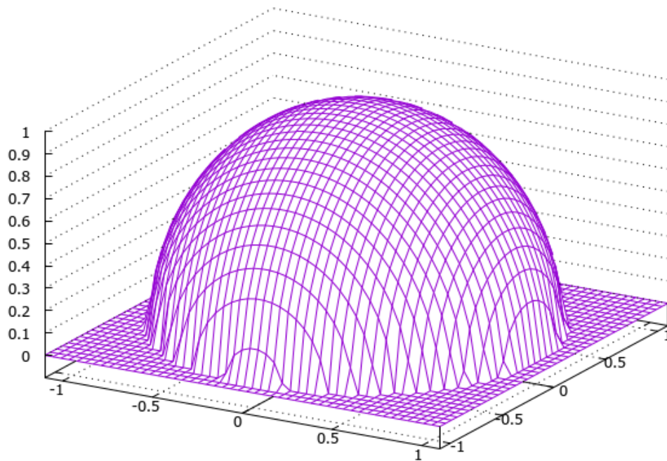
Рис. 11.1. Функция z = \sqrt{1 - x^2 - y^2} .
