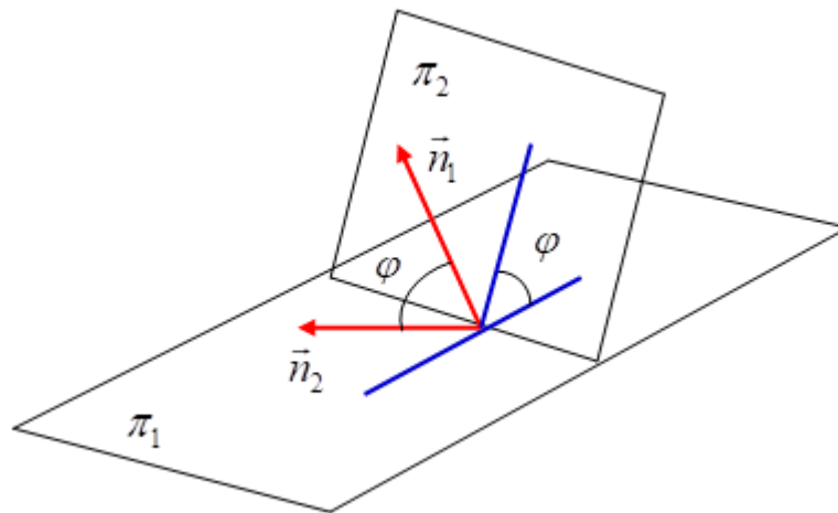
Рис. 4.5. Угол между плоскостями.
