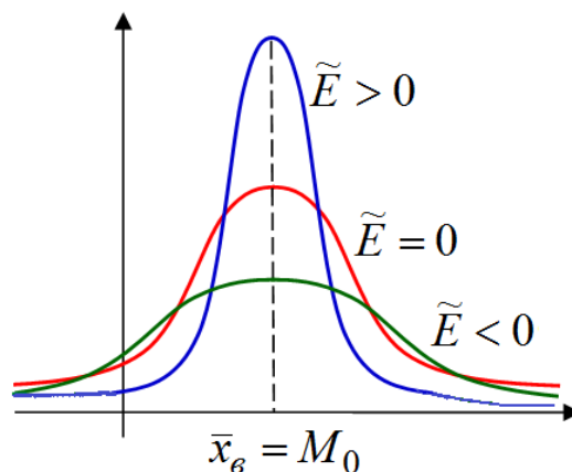
Рис. 18.5. Значения коэффициента эксцесса.
