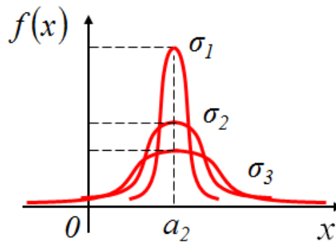
Рис. 17.8. Влияние параметра \sigma на форму нормальной кривой.
