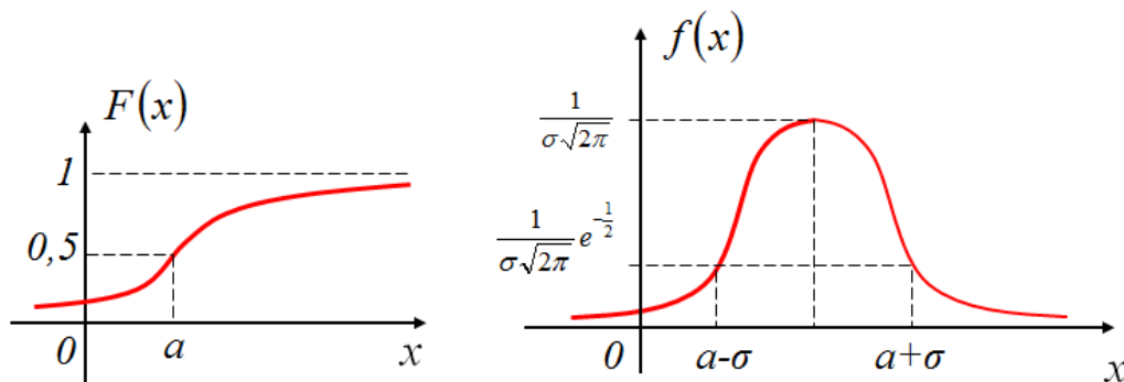
Рис. 17.6. Графики функции и плотности распределения случайной величины, распределенной по нормальному закону.
