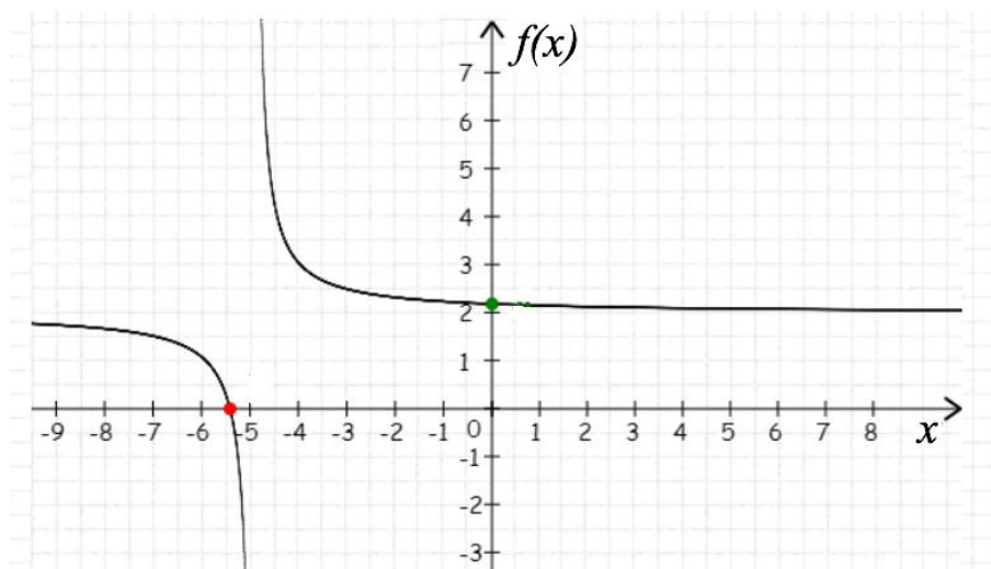
Рис. 9.11. График функции f(x) = 2 + \frac{1}{x+5} .
