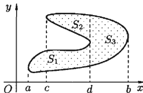
Рис. 12.6. Площадь фигуры, имеющей «сложную» конфигурацию.
