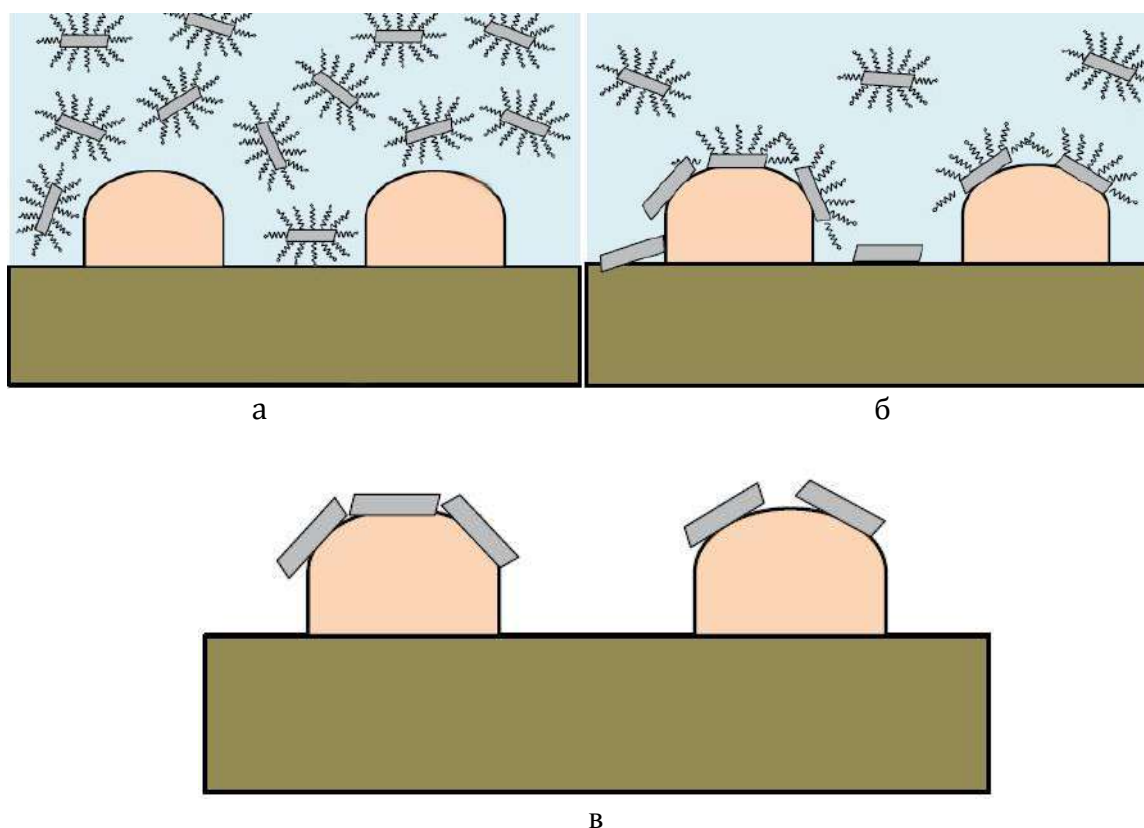
Рис. 7. Схематичное изображение механизма окрашивания следов рук мелкодисперсным проявителем: а – мицеллы, образованные ПАВ вокруг частиц дисульфида молибдена, в водной среде; б – осаждение и прикрепление частиц дисульфида молибдена к кожному жиру; в – папиллярные линии, окрашенные дисульфидом молибдена [3, с. 328]
