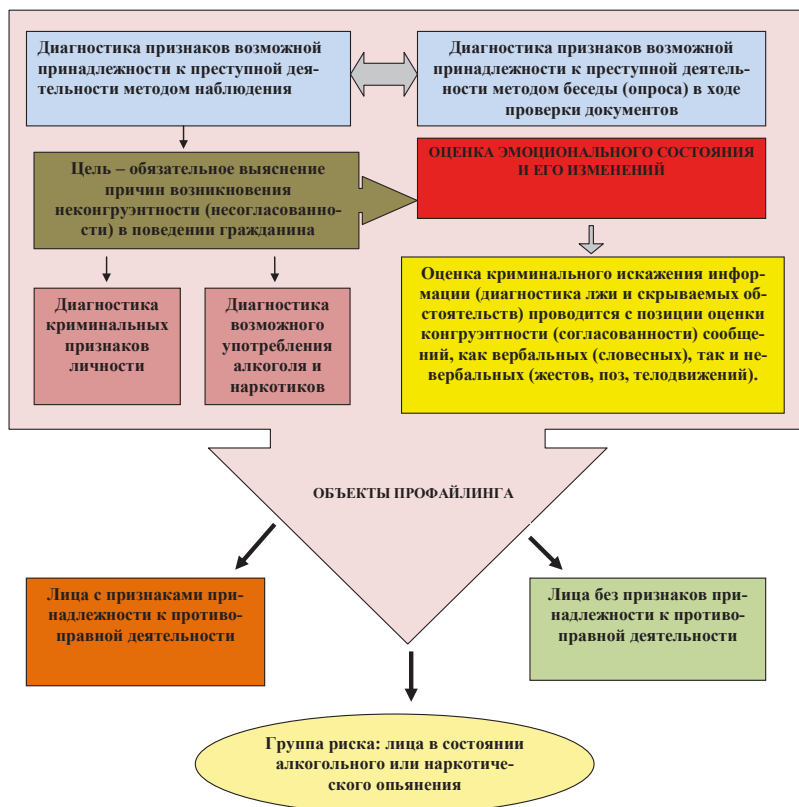
Рис. 1. Схема профайлинга
