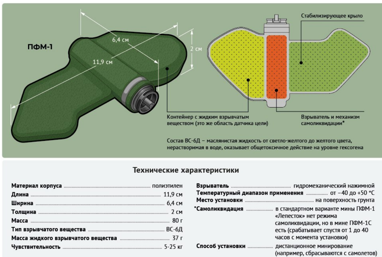
Рис. 1. Общее устройство и технические характеристики мины ПФМ-1 «Лепесток»
