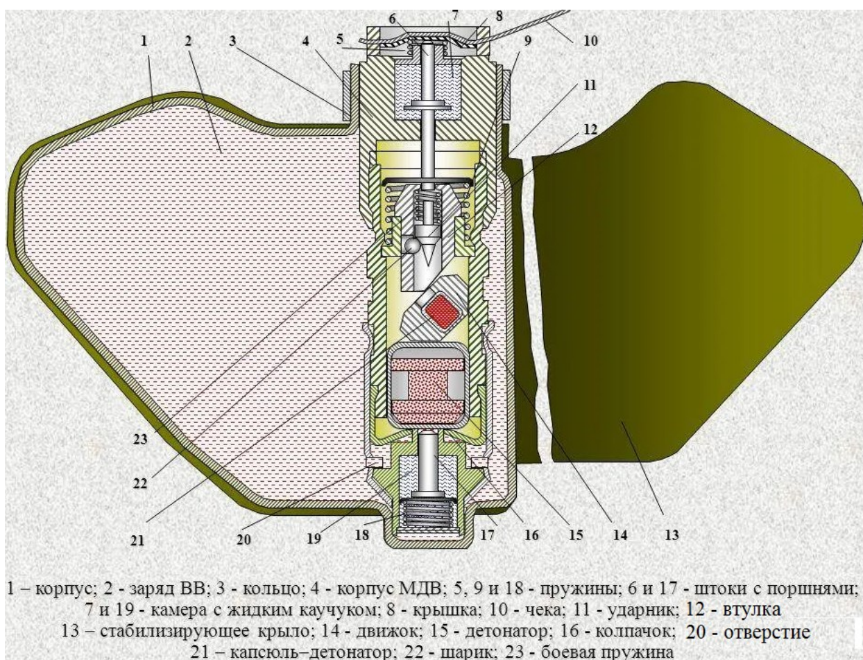
Рис. 2 Устройство мины ПФМ-1
