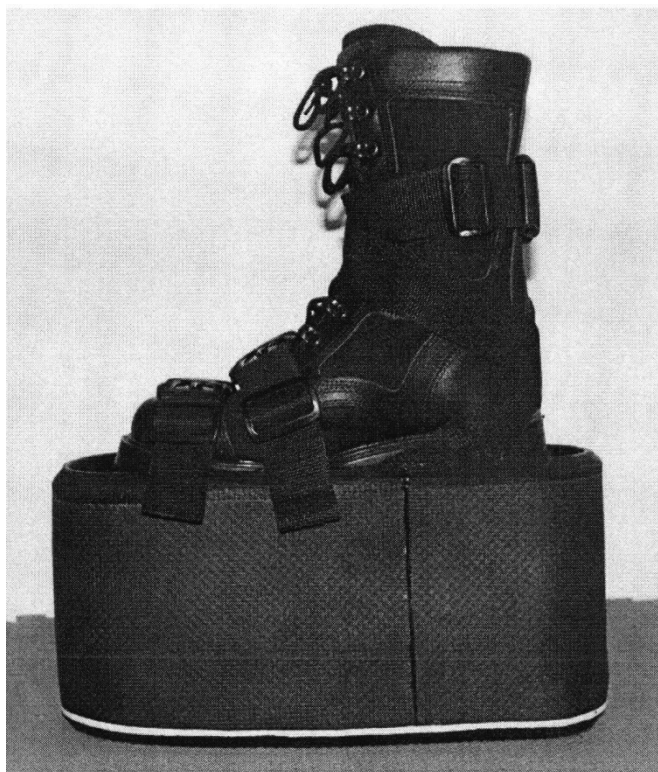
Рис. 7. Вариант взрывозащитной обуви на платформе.
