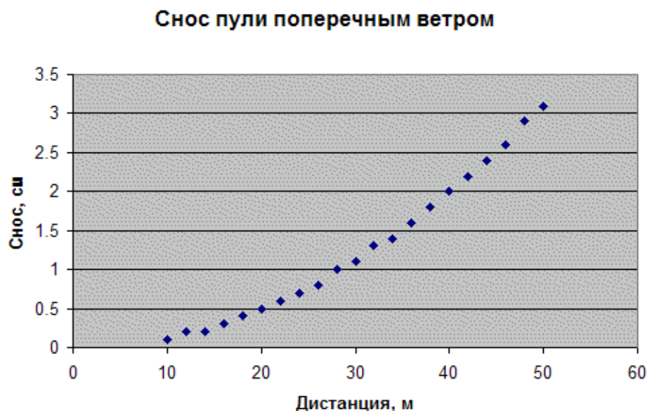
Рисунок – 1. Влияние ветра на полет пули
