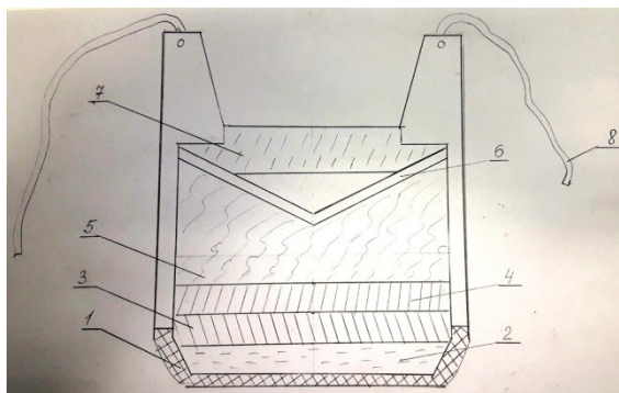
Рис. 7. Вариант взрывозащитной обуви на платформе.
