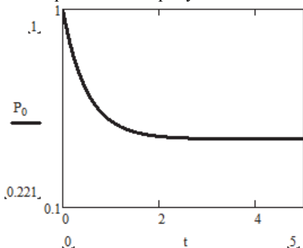
Рисунок 2. Вероятность состояния S_0
