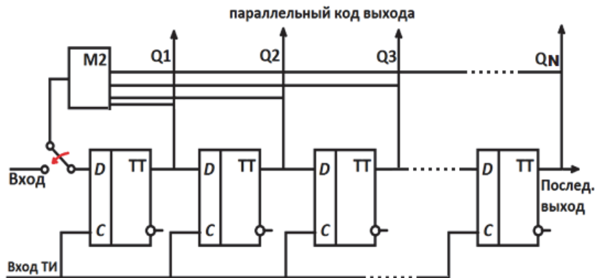
Рисунок 2. Функциональная схема линейного рекуррентного регистра
