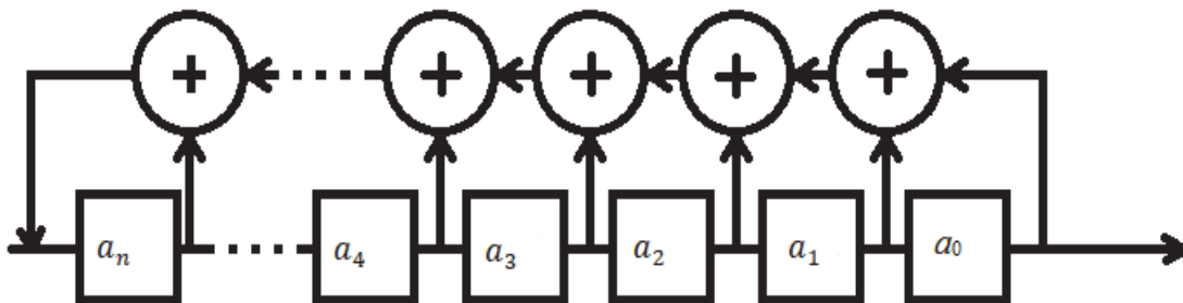
Рисунок 1. Структурная схема линейного регистра сдвига для многочлена степени n .
