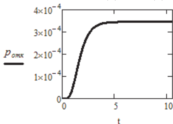
Рисунок 6. Вероятность отказа комплекса в обслуживании
