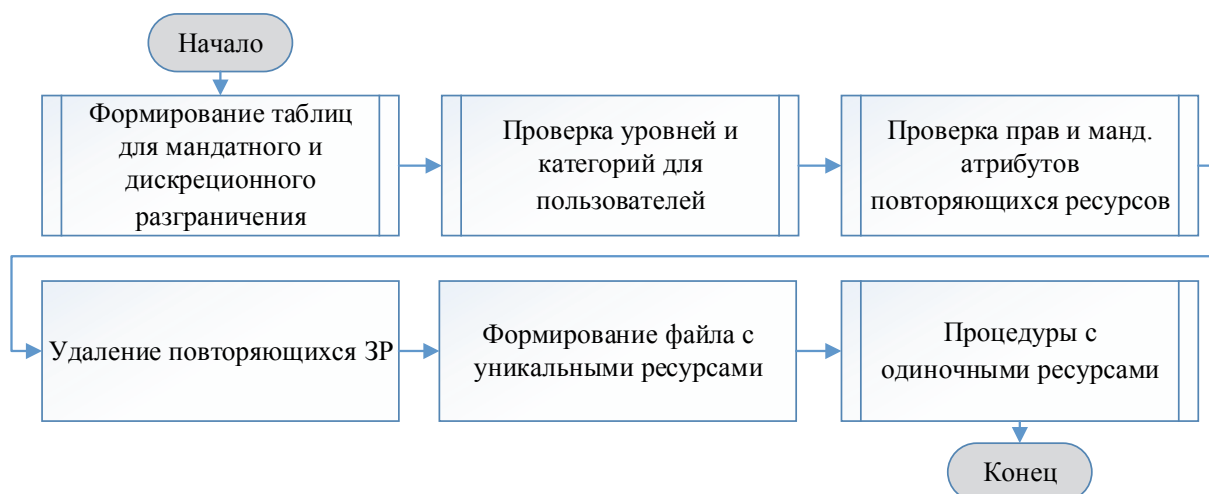
Рисунок 1. Общий алгоритм сравнения прав
