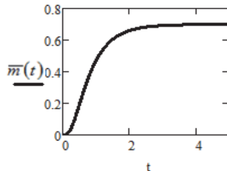
Рисунок 5. Среднее число криптограмм в очереди
