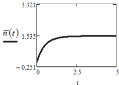
Рисунок 4. Среднее число занятых комплектов аппаратуры
