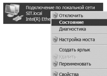
Рис. 6.16. Сетевое подключение
