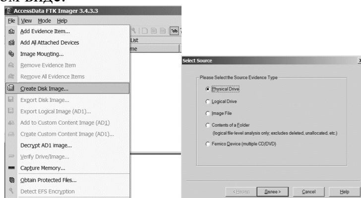
Рис. 6.4. Создание образа
