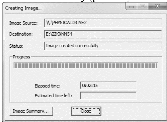
Рис. 6.9. Создание образа
