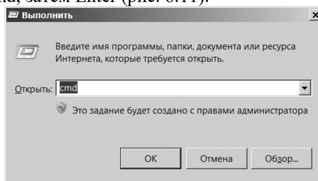
Рис. 6.11. Окно «Выполнить»
