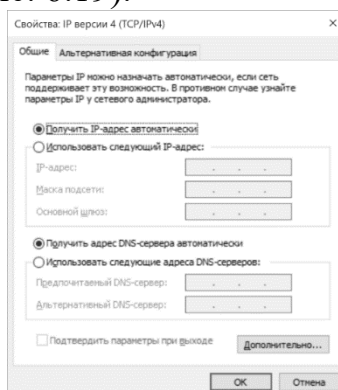
Рис. 6.19. Свойства IPv4
