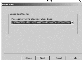
Рис. 6.5. Устройство – источник
