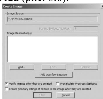
Рис. 6.6. Создание образа
