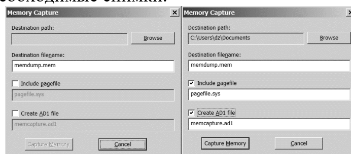
Рис. 6.3. Настройки снимка
