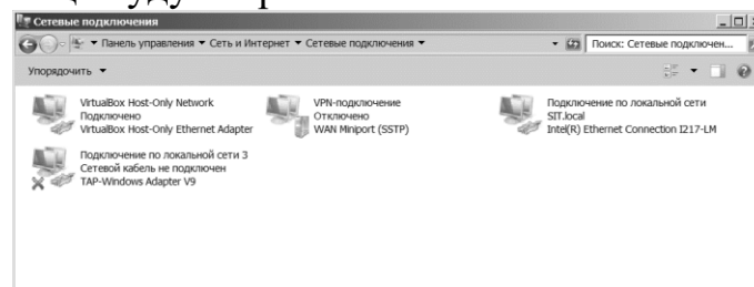
Рис. 6.15. Сетевые подключения
