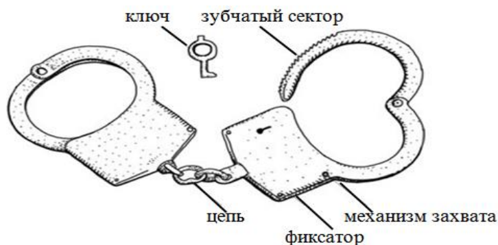
Рис. 13. Общая конструкция современных наручников
